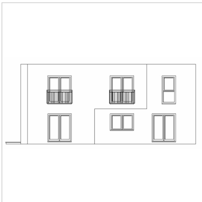
Modern Duo 14 - A3
